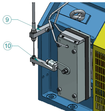
图 21 松闸机构
