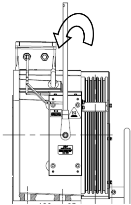
图 13 松闸手柄链接示意图
