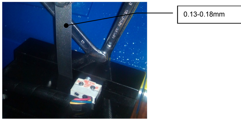
图 11 间隙值
