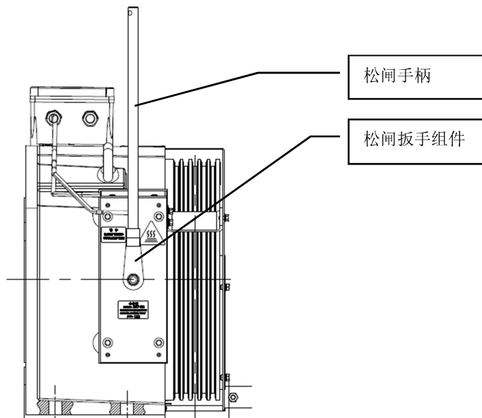
图 12 手动松闸装置图示
