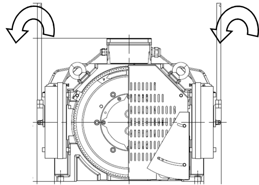
图 14 松闸手柄使用示意图
