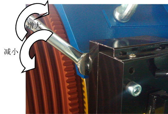
图 5 转动空心螺栓示意图
