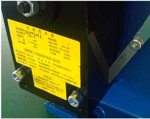
图 8 对角间隙
