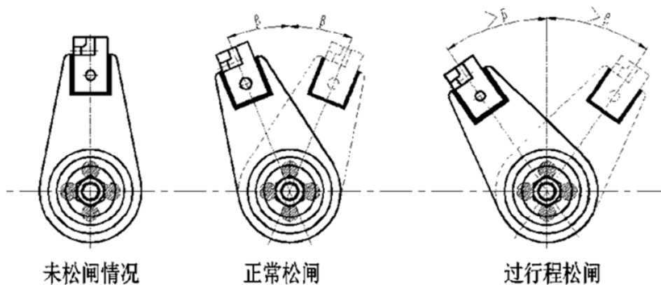
图 15 松闸角度示意图
