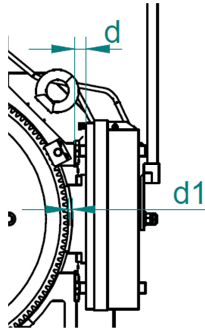
图 28 动板面与框架安装面距离 d 或刹车片厚度 d_1
