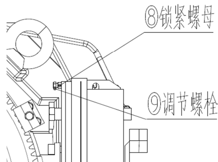
图 2 制动器外观
