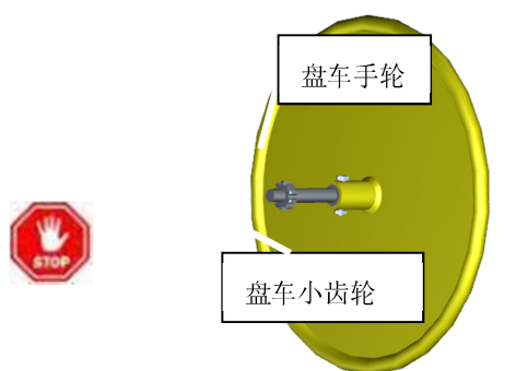
图 16 拧松链接螺栓
